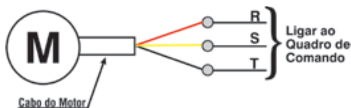
Esquema de ligação dos motores trifásicos com 01 cabo chato.
