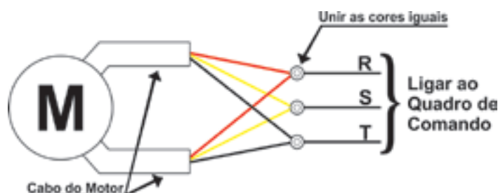
Esquema de ligação dos motores trifásicos com 01 cabo chato.
